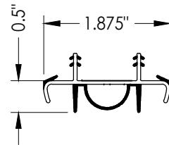
8 DOOR BOTTOM SWEEP (Articulating)
